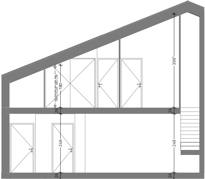
COUPE AA
