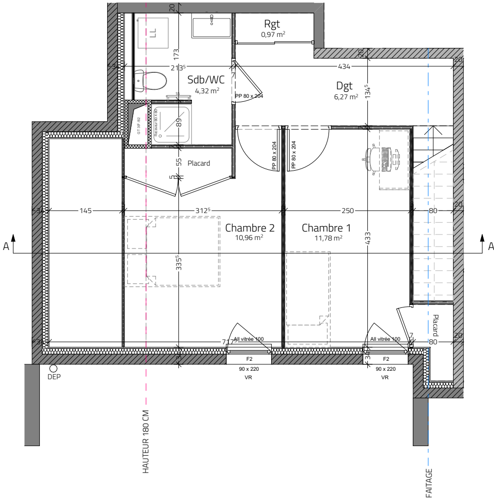
Niveau +1
